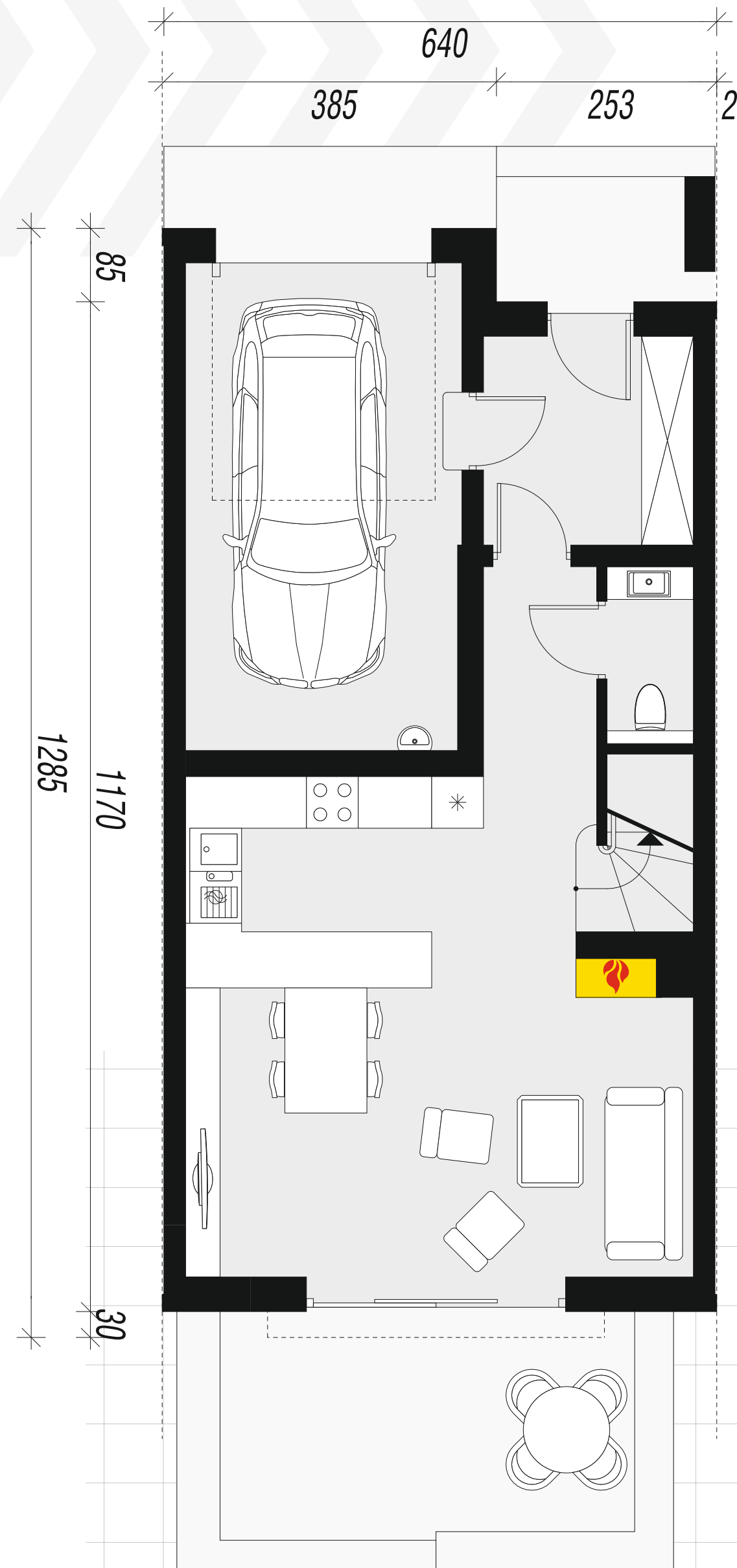
rzut parteru
