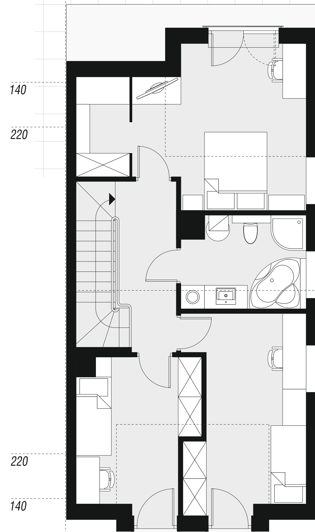
rzut poddasza
