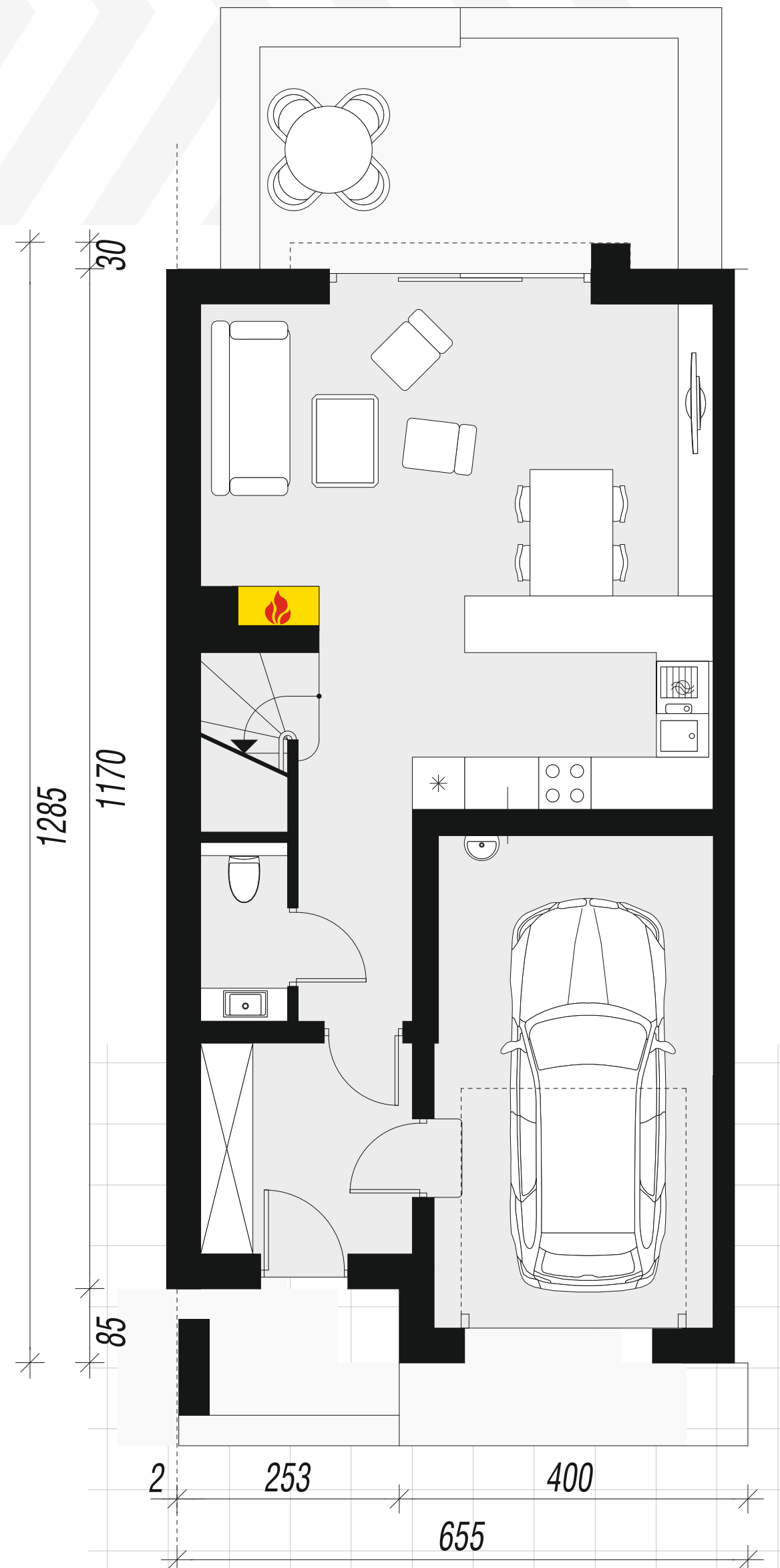
rzut parteru
