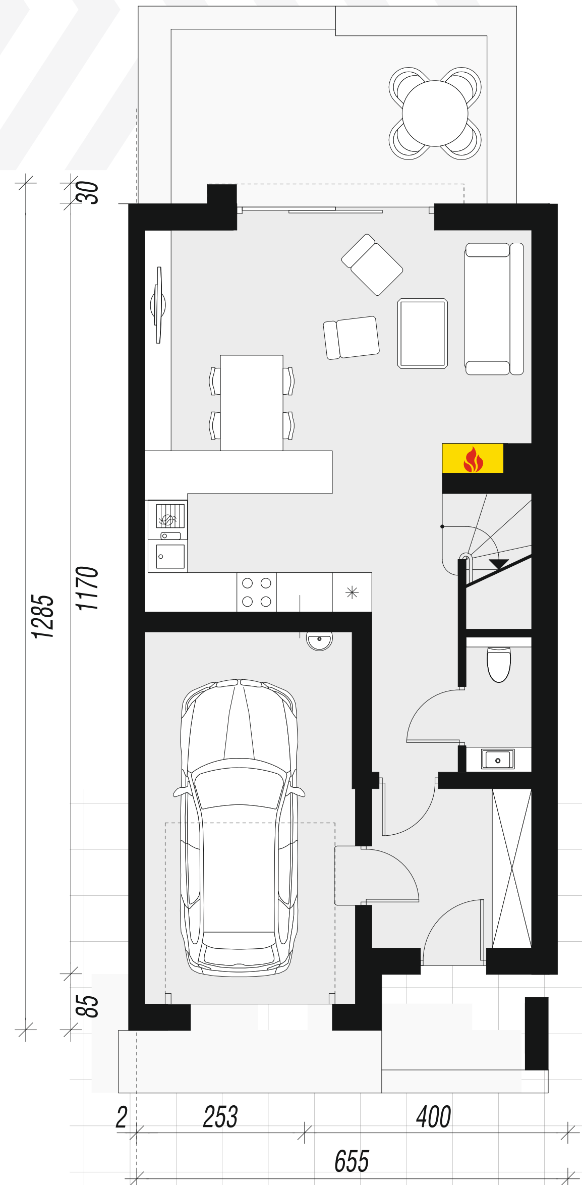
rzut parteru
